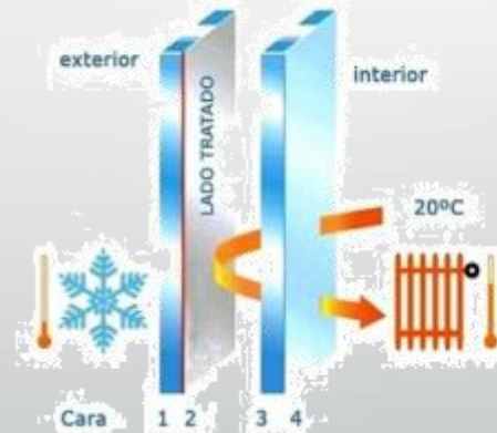
en invierno, mayor retención del calor
